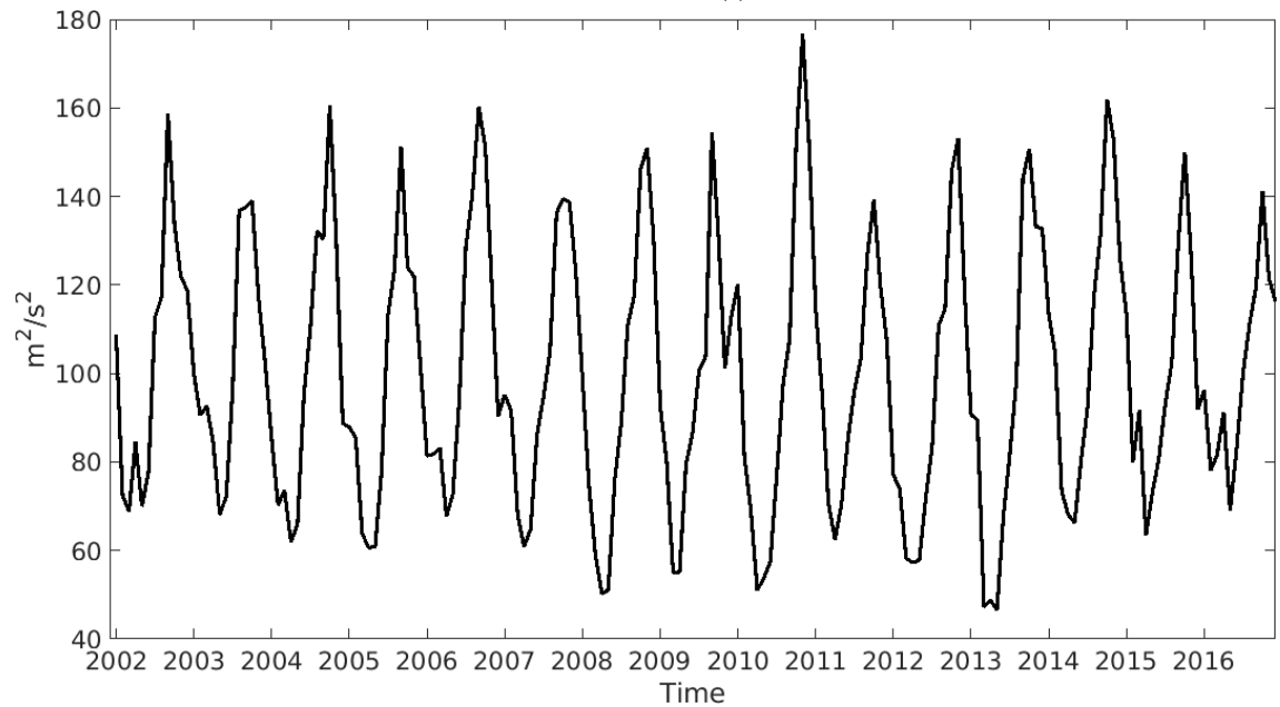
HighRes (b)
