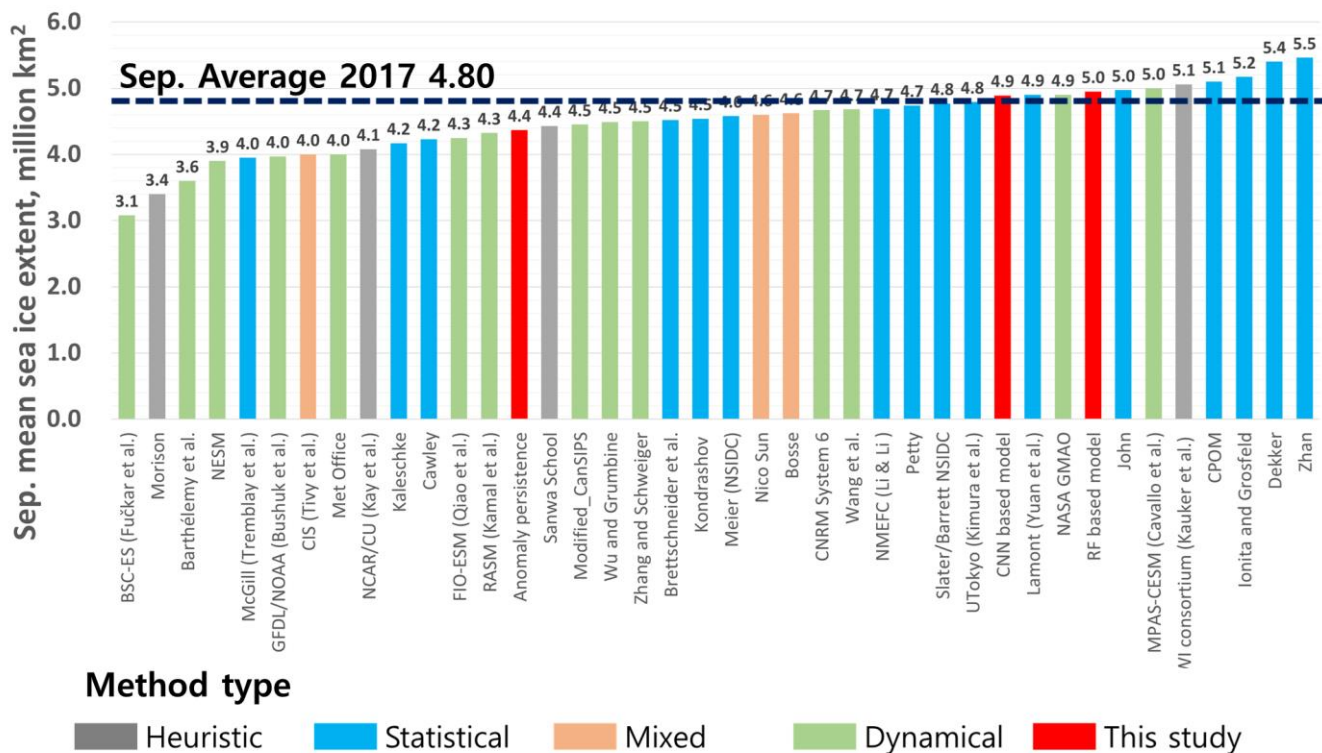
(d) Distribution of SIOs for September 2017 extent (August report)
