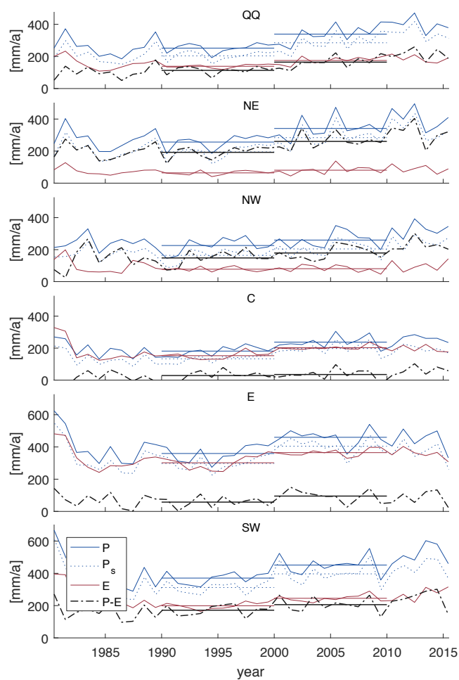
(b) MERRA-2
