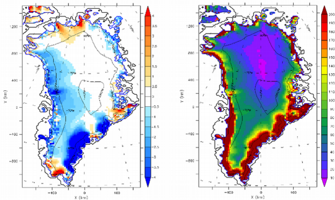
SMB trend over 1976-2014 (mmWE/yr 2 )
