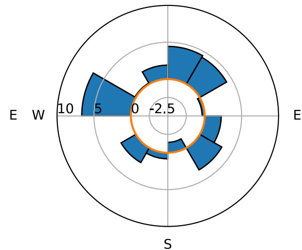
(d) P19: Jan. 15th N
