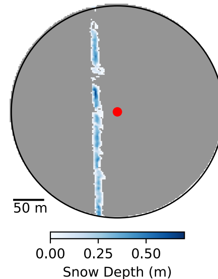
(h) P19: Jan. 15th - lidar DSM
