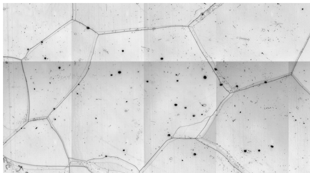
(d) 2872 m: impurity-poor ice (interglacial)
