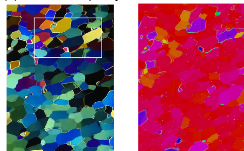
(d) 2872 m: impurity-poor ice (interglacial)
