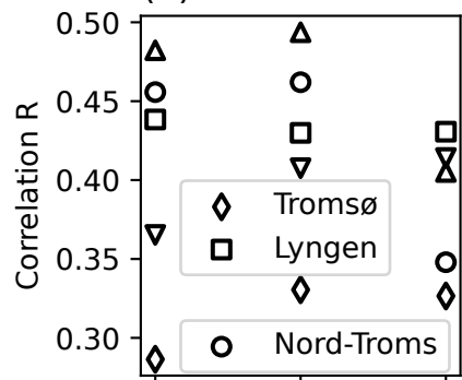
(d) ADF & AO Corr
