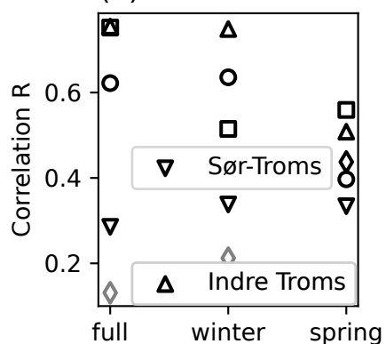
(d) ADF & AO Corr
