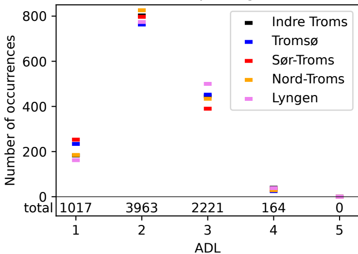
(a) ADL per region
