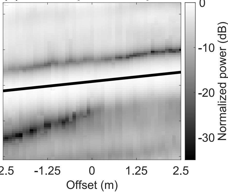
(d) LO-SAR-processed power
