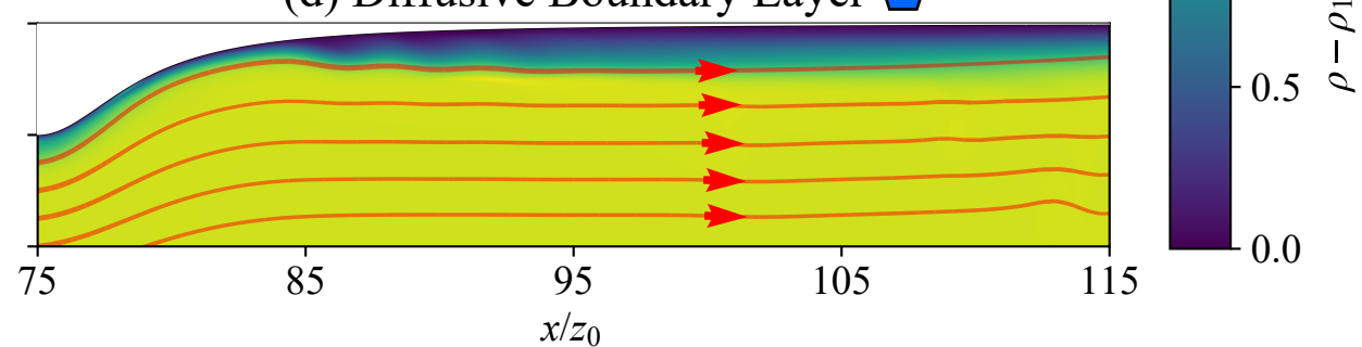
(d) Diffusive Boundary Layer ◆
