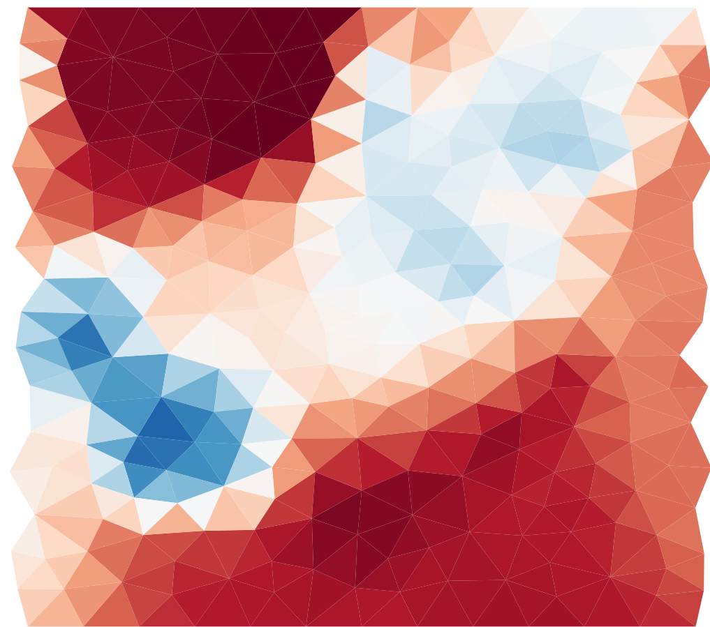
(d) \text{Corr}(v, \alpha) day 18
