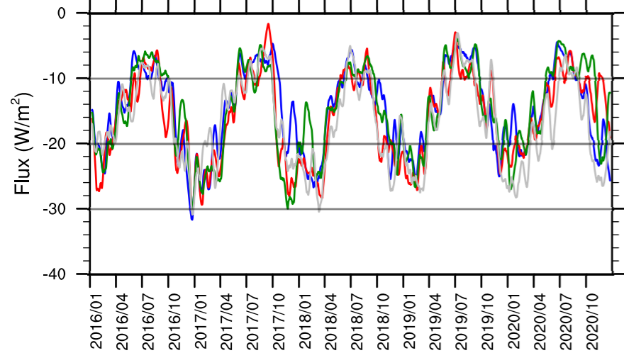
(d) Net longwave flux
