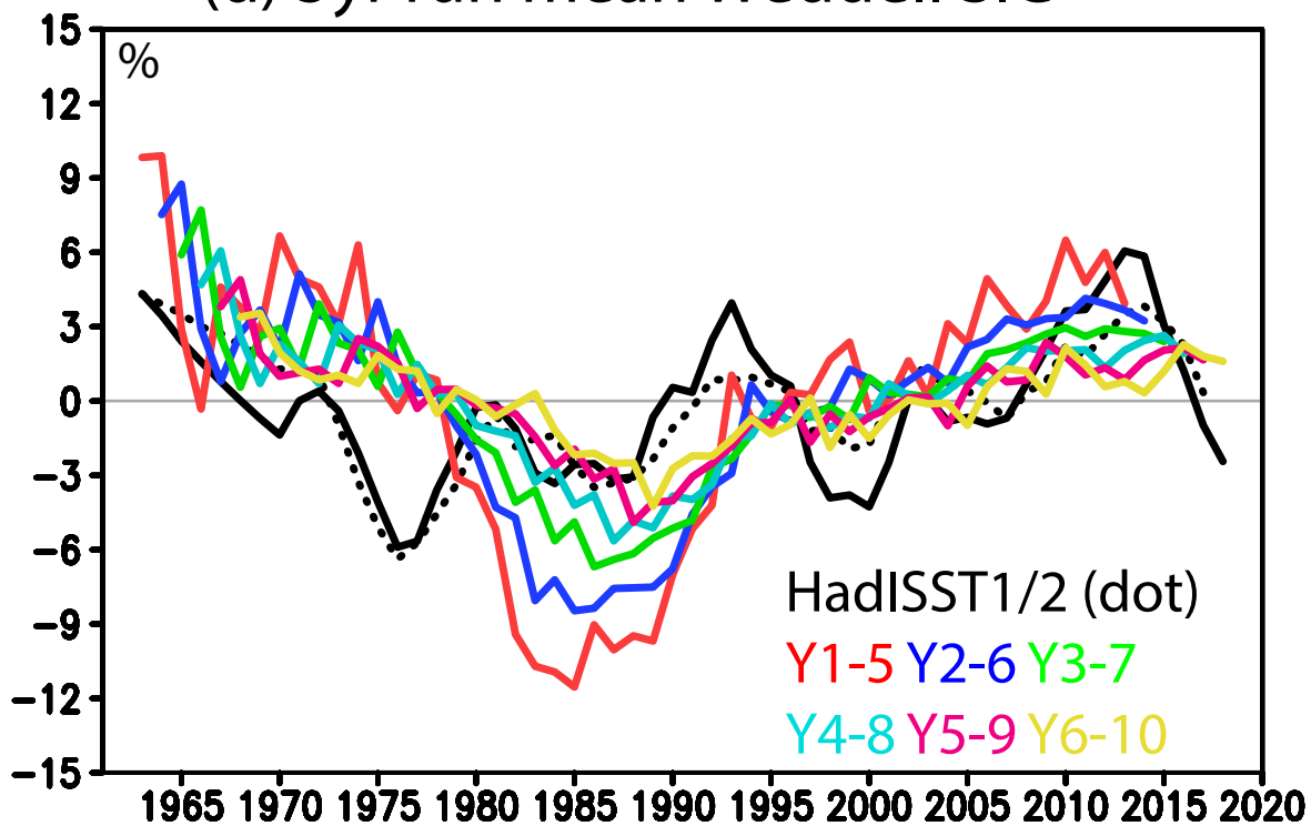
(d) 5yr run mean Weddell SIC
