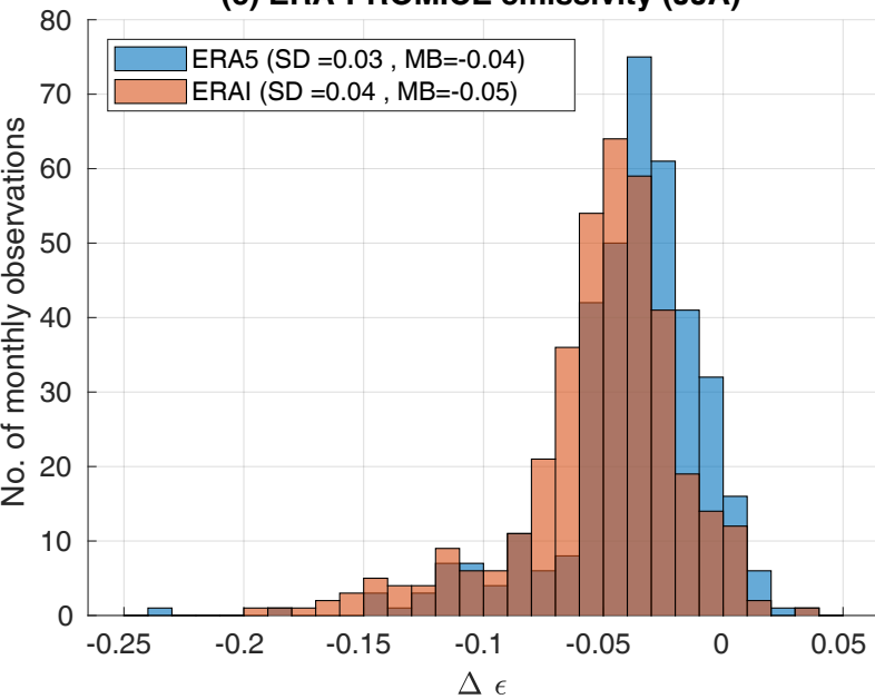
(c) ERA-PROMICE emissivity (JJA)
