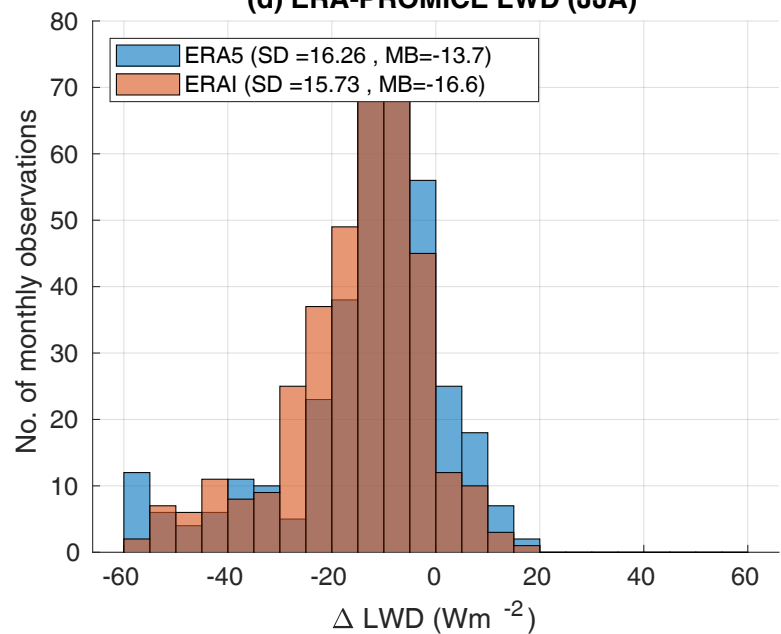
(d) ERA-PROMICE LWD (JJA)
