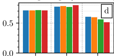
Surf. precip. / Valid sig.
