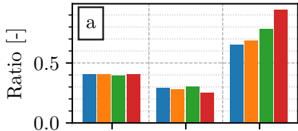
Virga / Valid sig.
