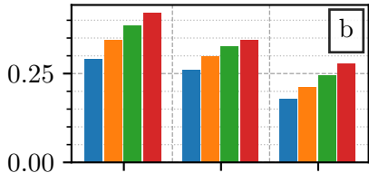
Surf. precip. / Valid sig.
