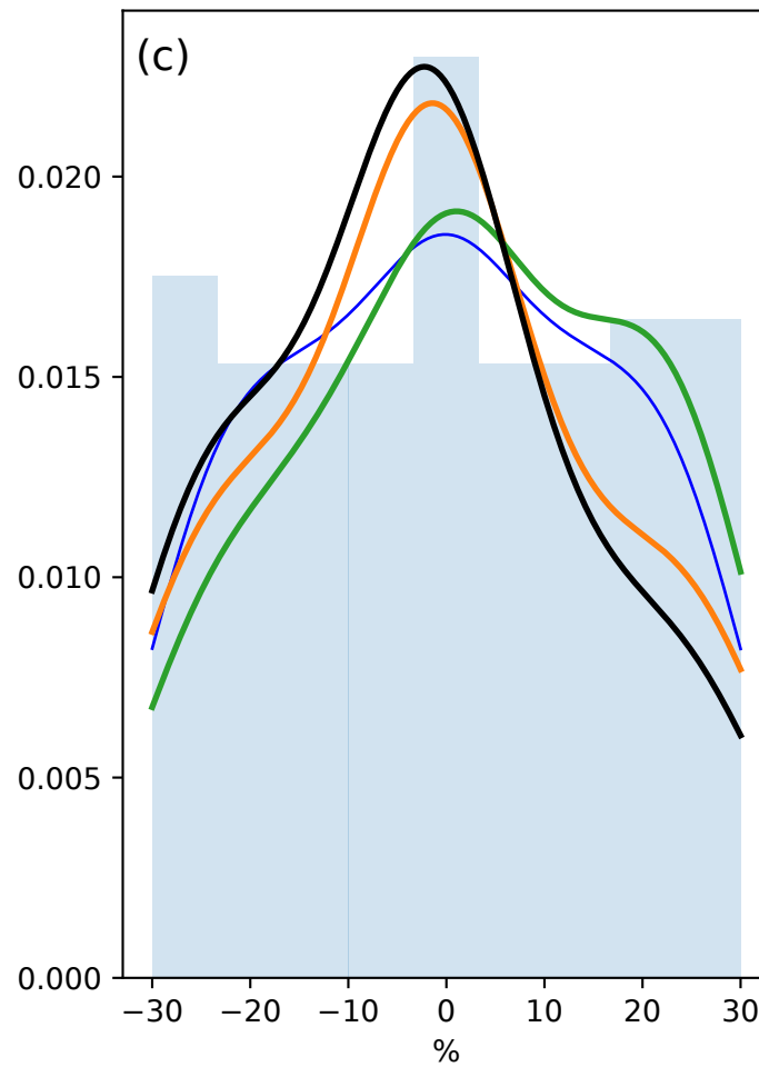
SMB mean shift
