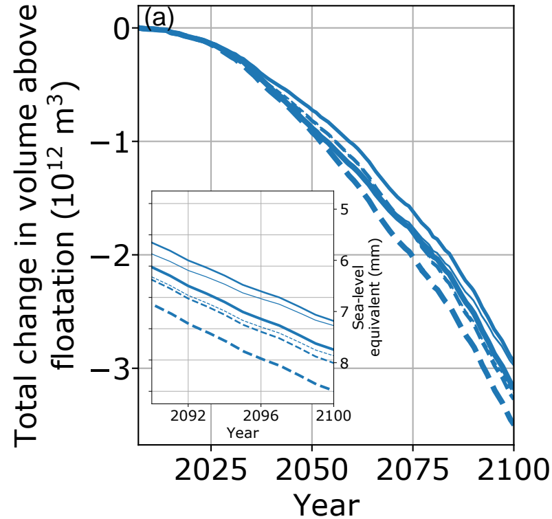
HadGEM2
