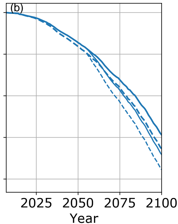
HadGEM2
