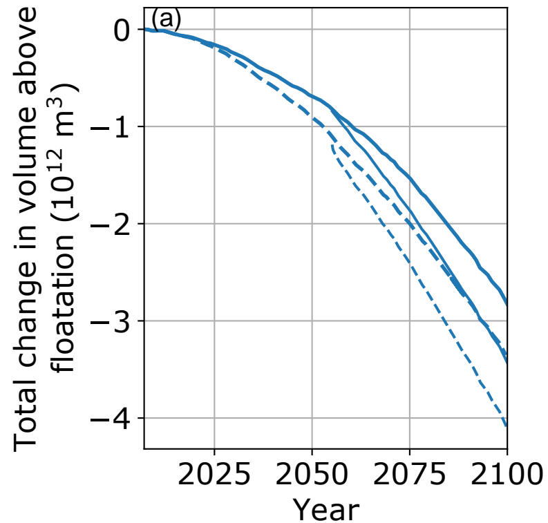
MIROC5
