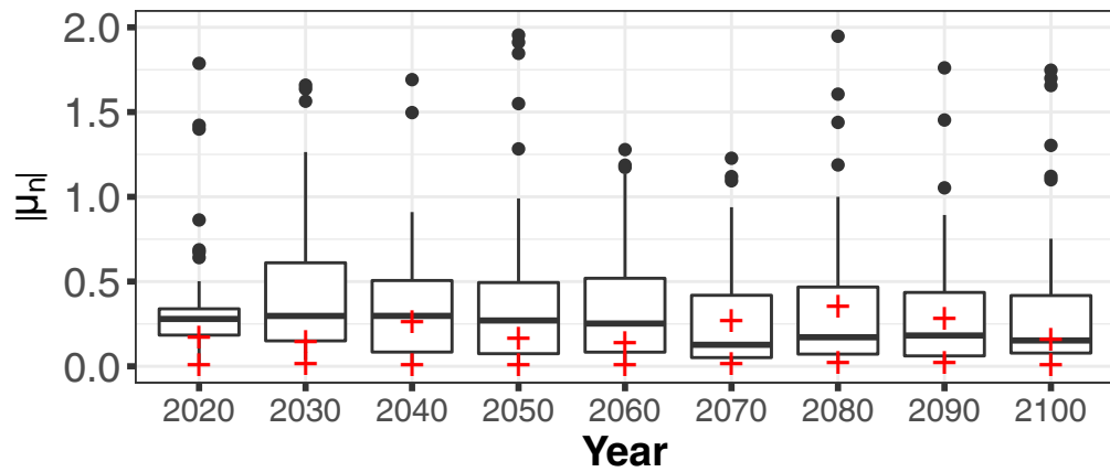
(d) Numerics
