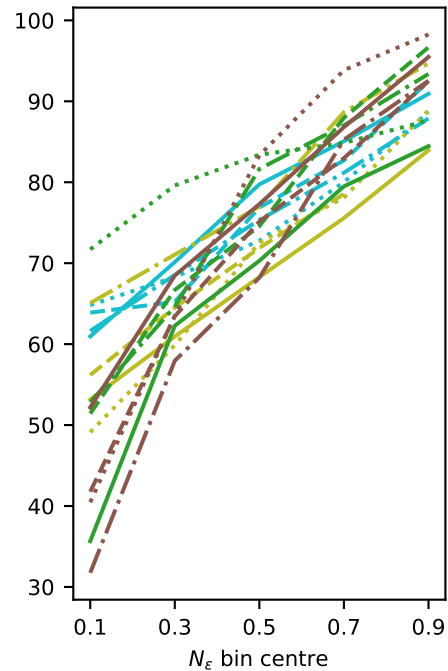
(d) RH
