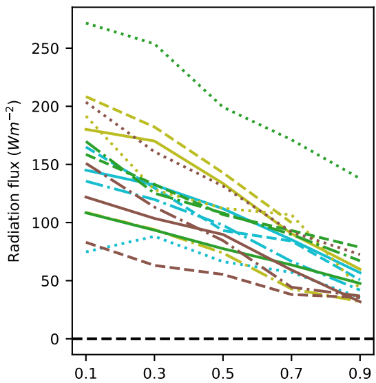
(d) SWnet cloud effect
