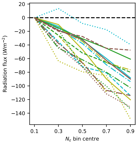
(d) SWnet cloud effect
