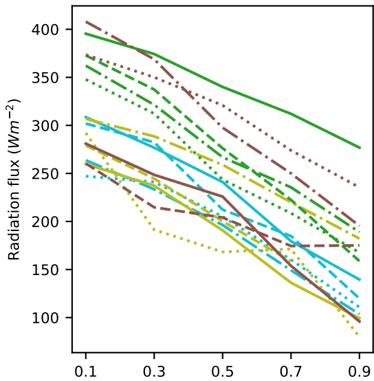
(d) SWin cloud effect
