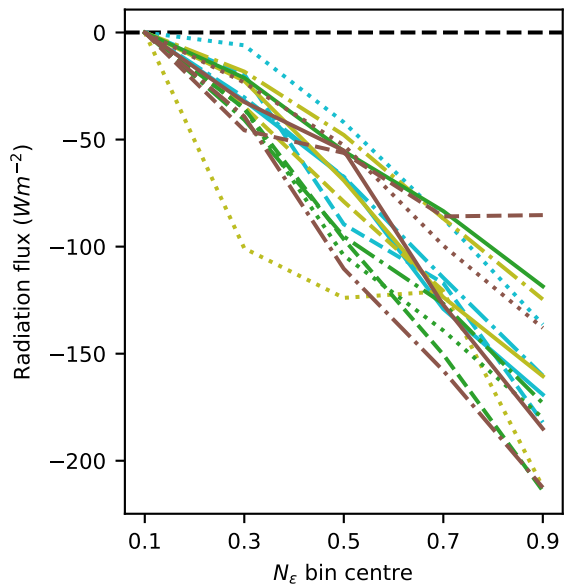
(d) SWin cloud effect
