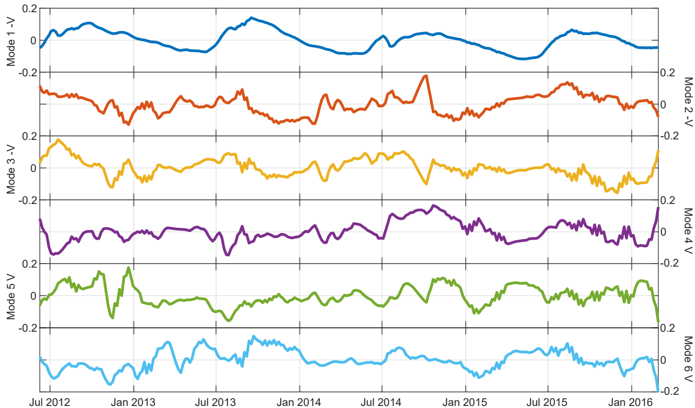
(d) POD temporal coefficients
