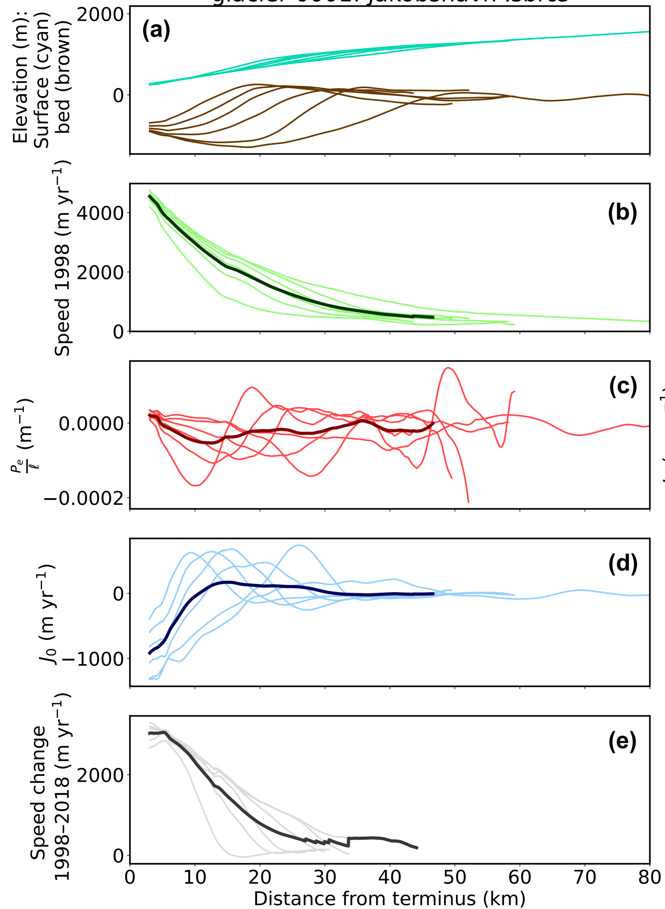
glacier 0001: Jakobshavn Isbræ
