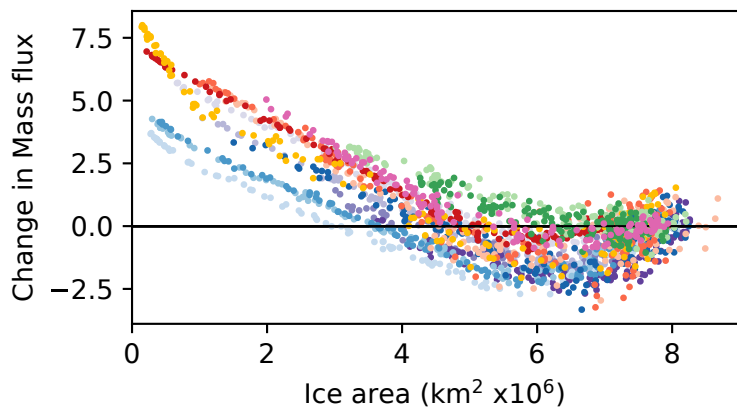
(d) Basal melt
