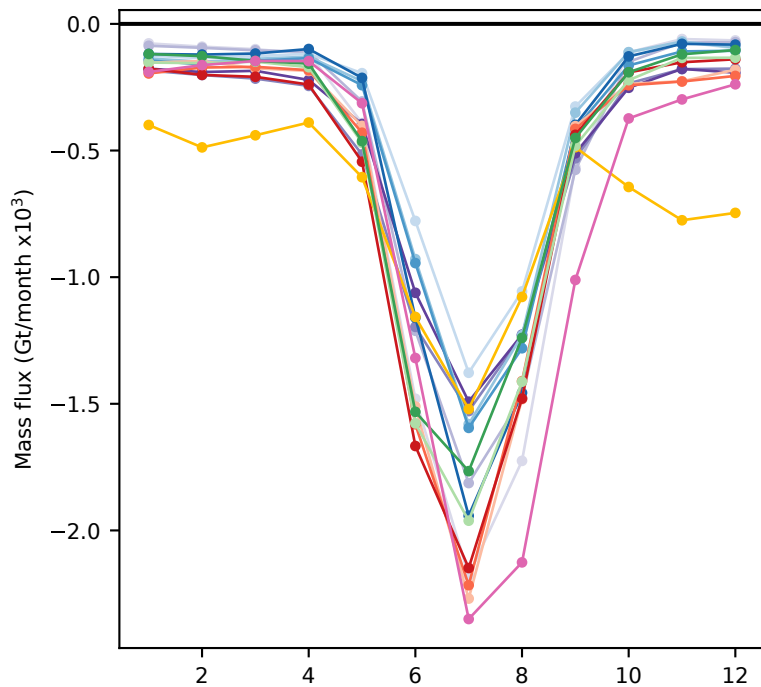
(d) Basal melt
