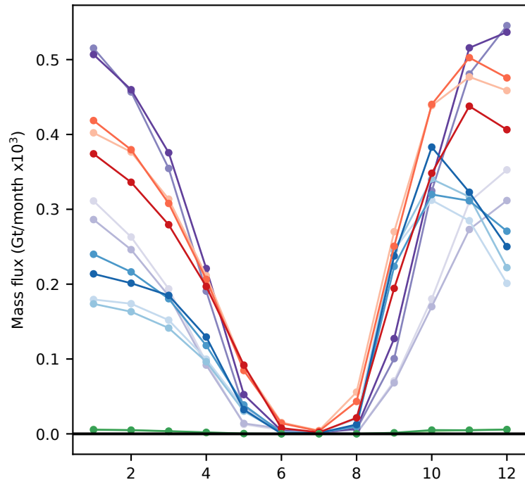
(d) Basal melt
