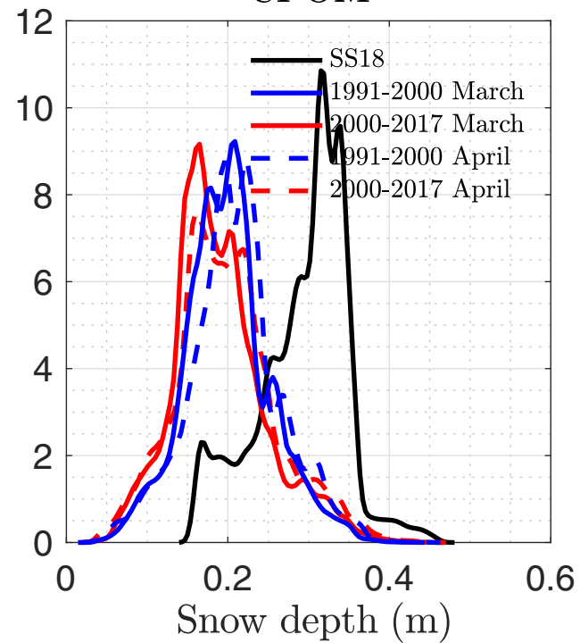
CPOM
