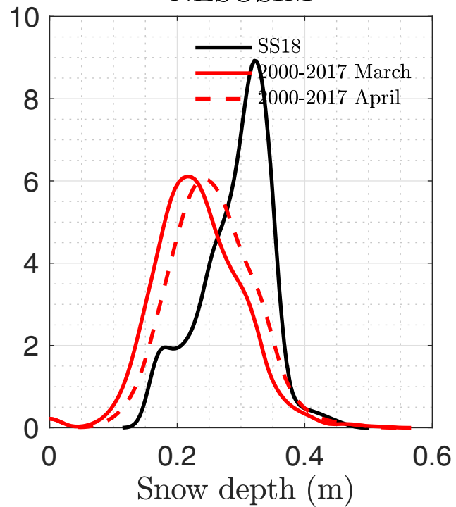
NESOSIM
