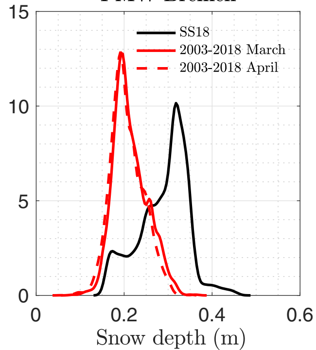
PMW Bremen
