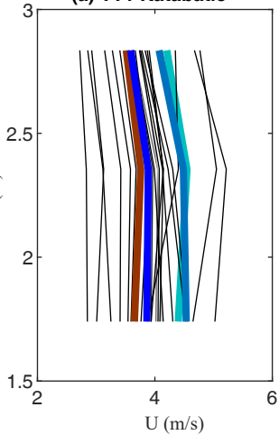
(a) TT1 Katabatic
