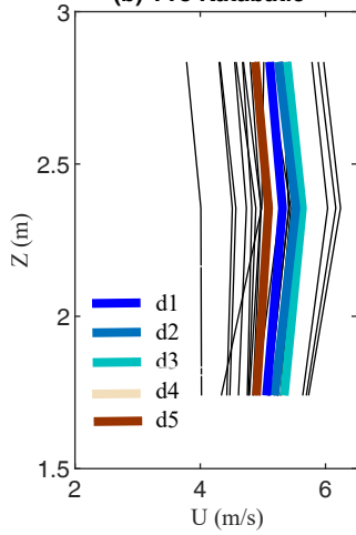
(b) TT3 Katabatic
