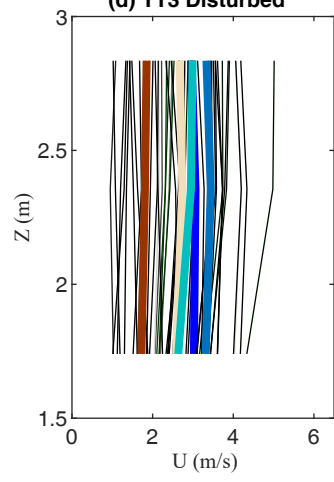
(d) TT3 Disturbed
