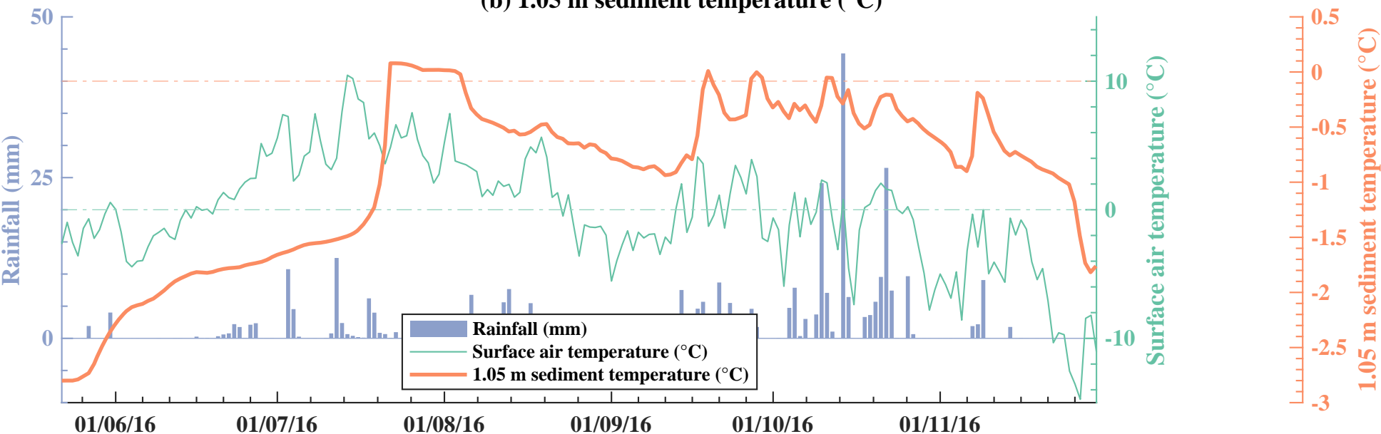
(b) 1.05 m sediment temperature (°C)
