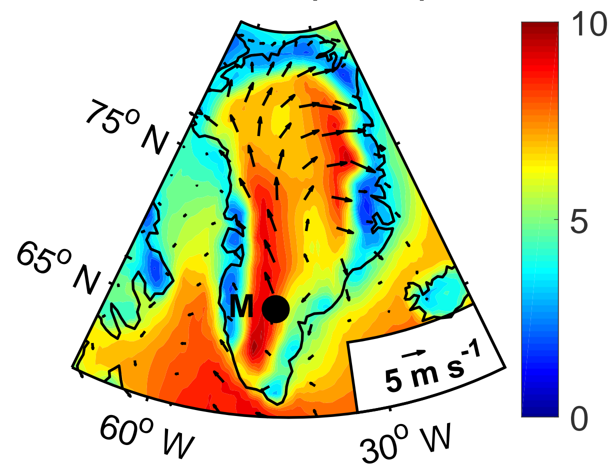
(a) SPD ( \text{m s}^{-1} )
