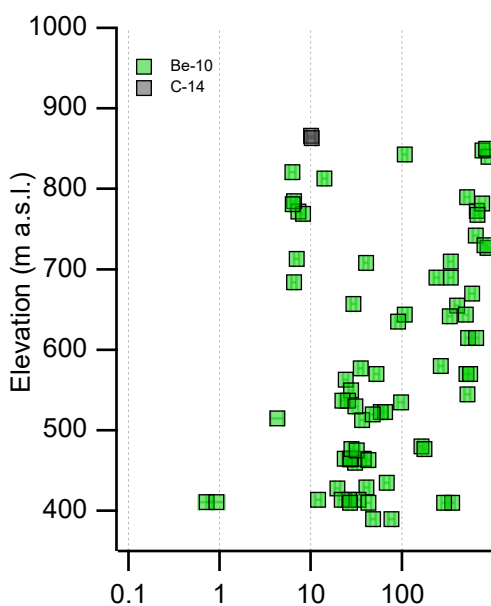
(b) Age (ka)
