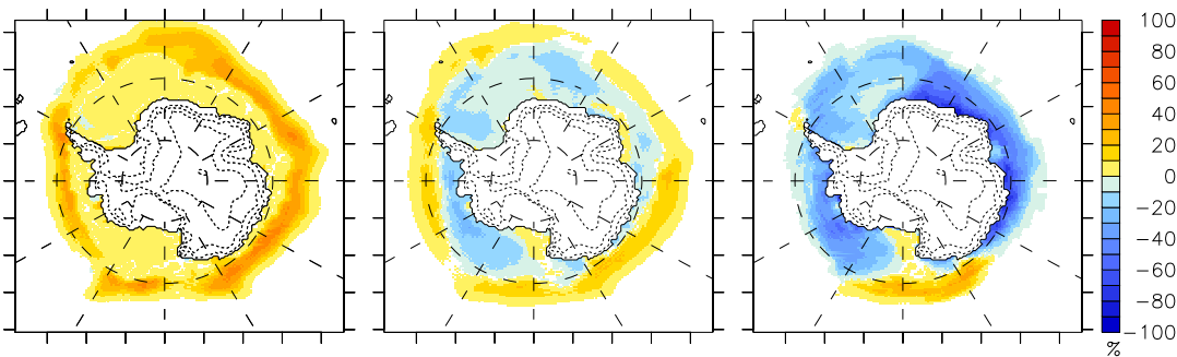
(d) SIC(NorESM1-ME)
