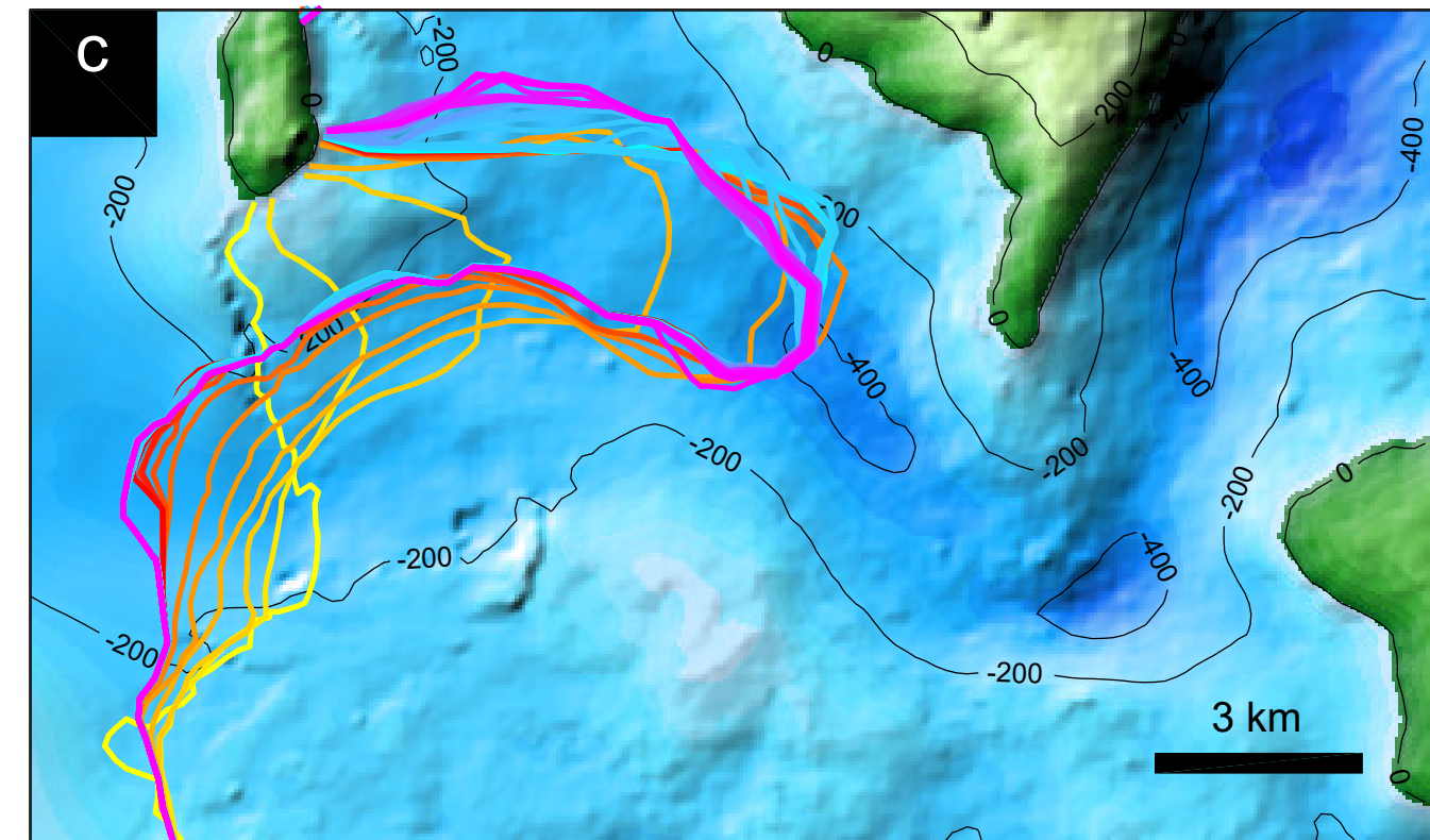
Eigencalving (EC)
