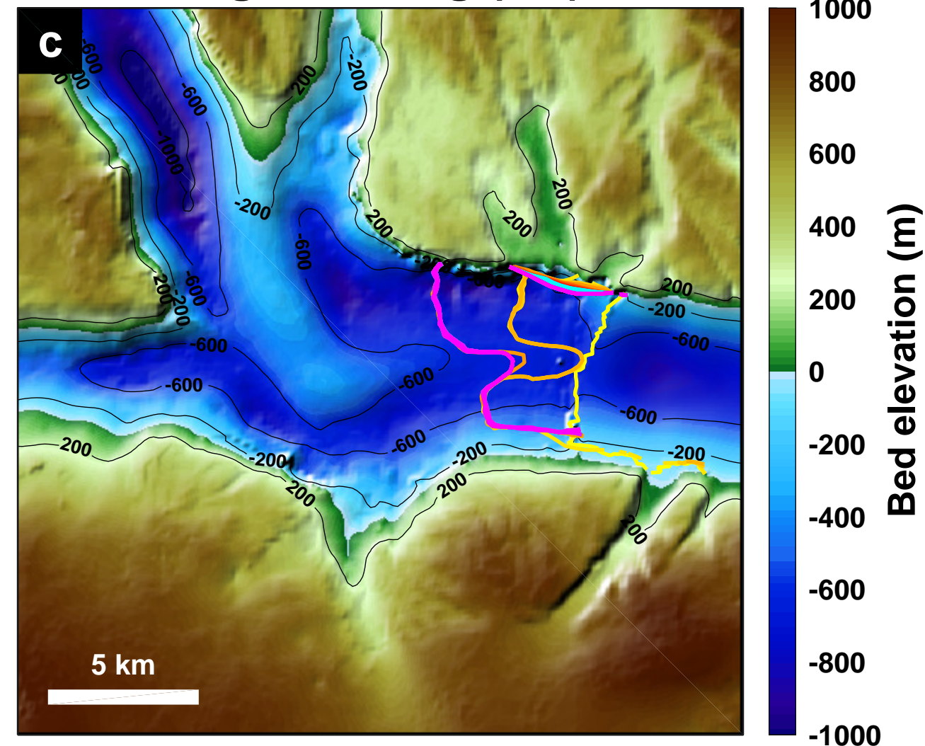
Eigencalving (EC)
