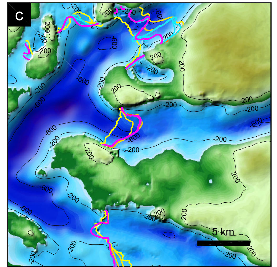
Eigencalving (EC)
