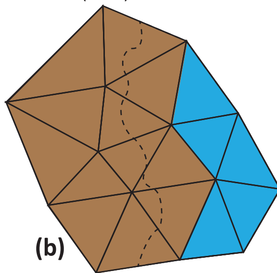
No melt parameterization (NMP)
