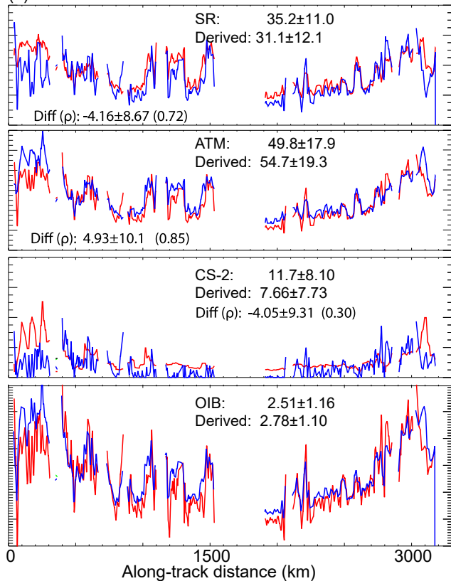
(b) 2011 Oct 25
