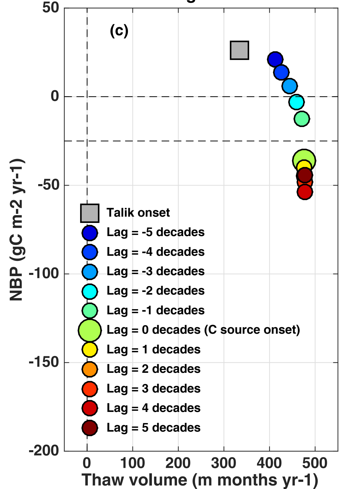
C source lags talik: fires
